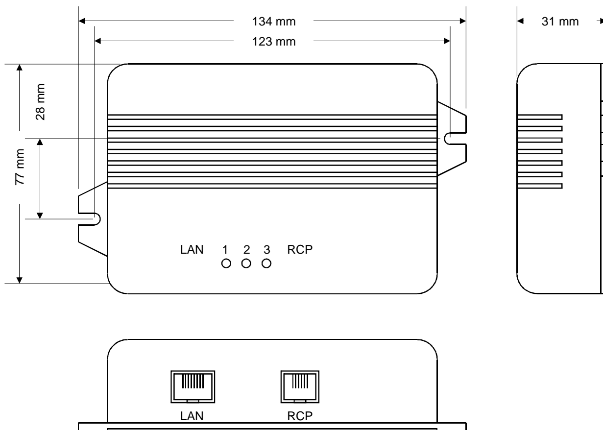
Rysunek 10: Konwerter sieciowy RCP48LS - wymiary główne
