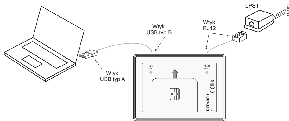
rys2. podłączenia konwertera RCP48CU
