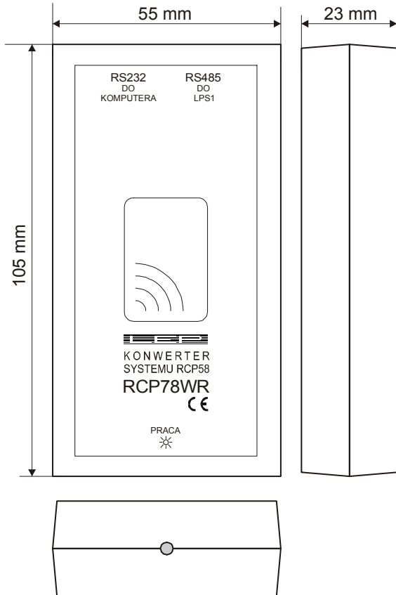
rys1. Konwerter RCP78WR - wymiary główne
