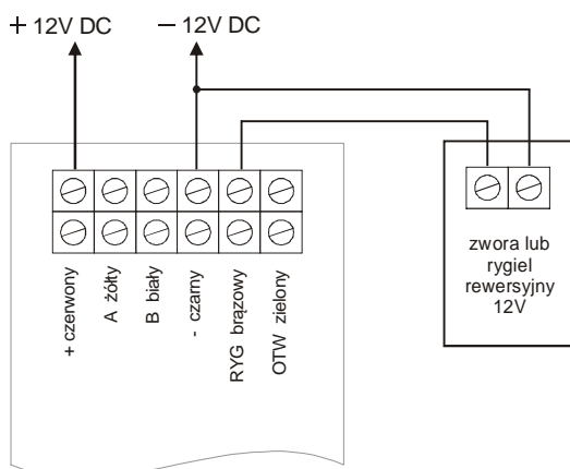
Rys.8a Podłączenie rygła rewersyjnego sterowanego jednym czytnikiem RCP78AR
