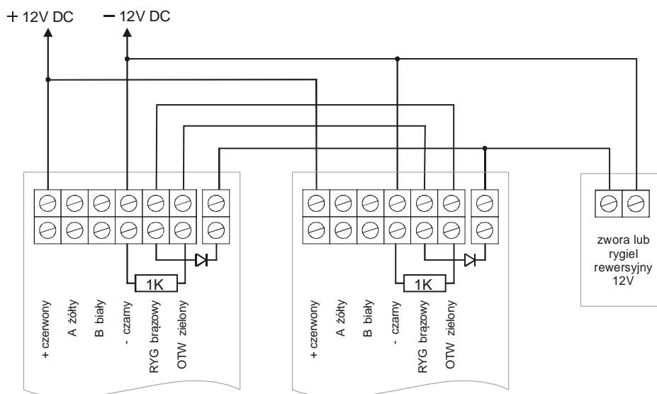
Rys.8b Podłączenie rygła rewersyjnego sterowanego dwoma czytnikami RCP78AR bez podłączonych przycisków OTW
