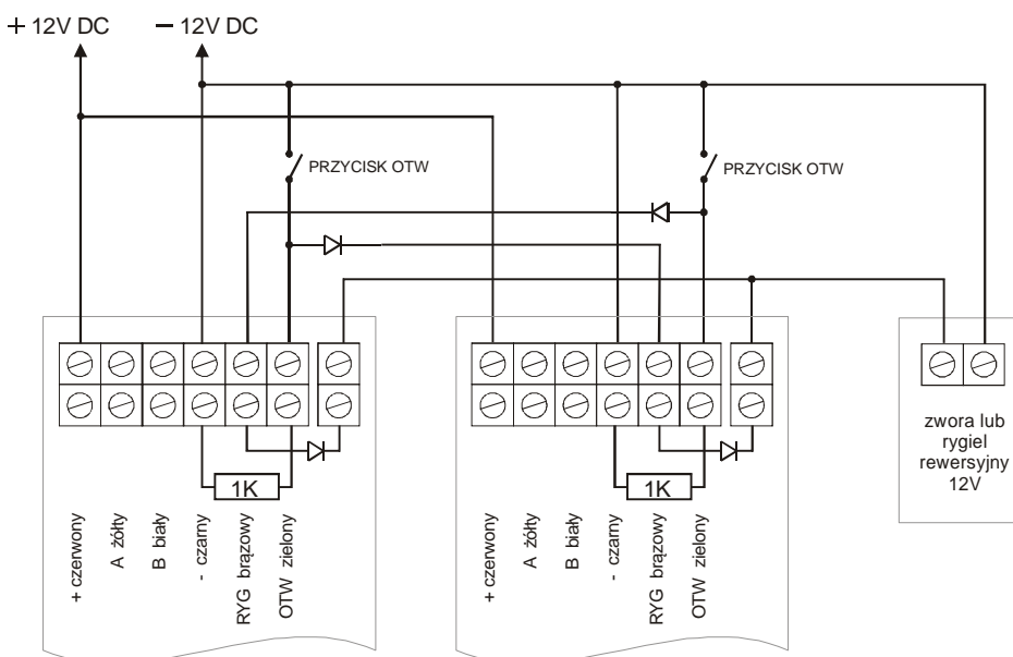
Rys.8c Podłączenie rygła rewersyjnego sterowanego dwoma czytnikami RCP78AR z podłączonymi przyciskami OTW
