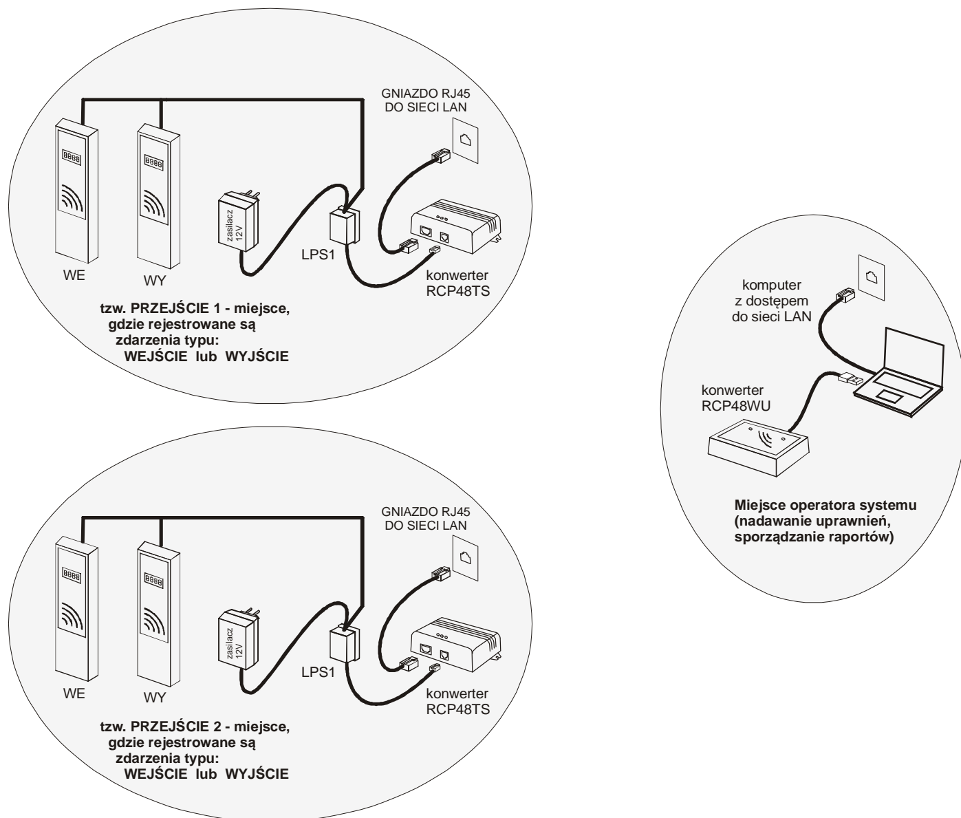
Rysunek 12: Przykładowy schemat struktury systemu (2 odrębne lokalizacje czytników)
