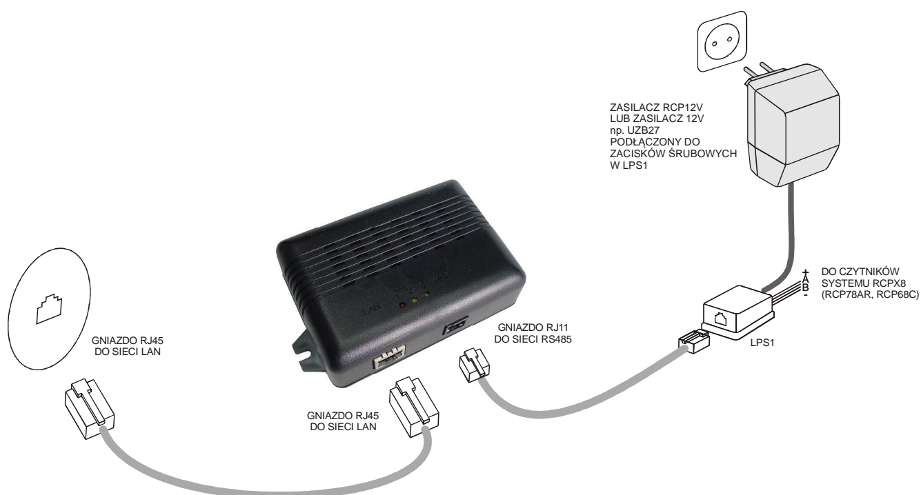
Rysunek 11: Podłączenie konwertera sieciowego RCP48TS
