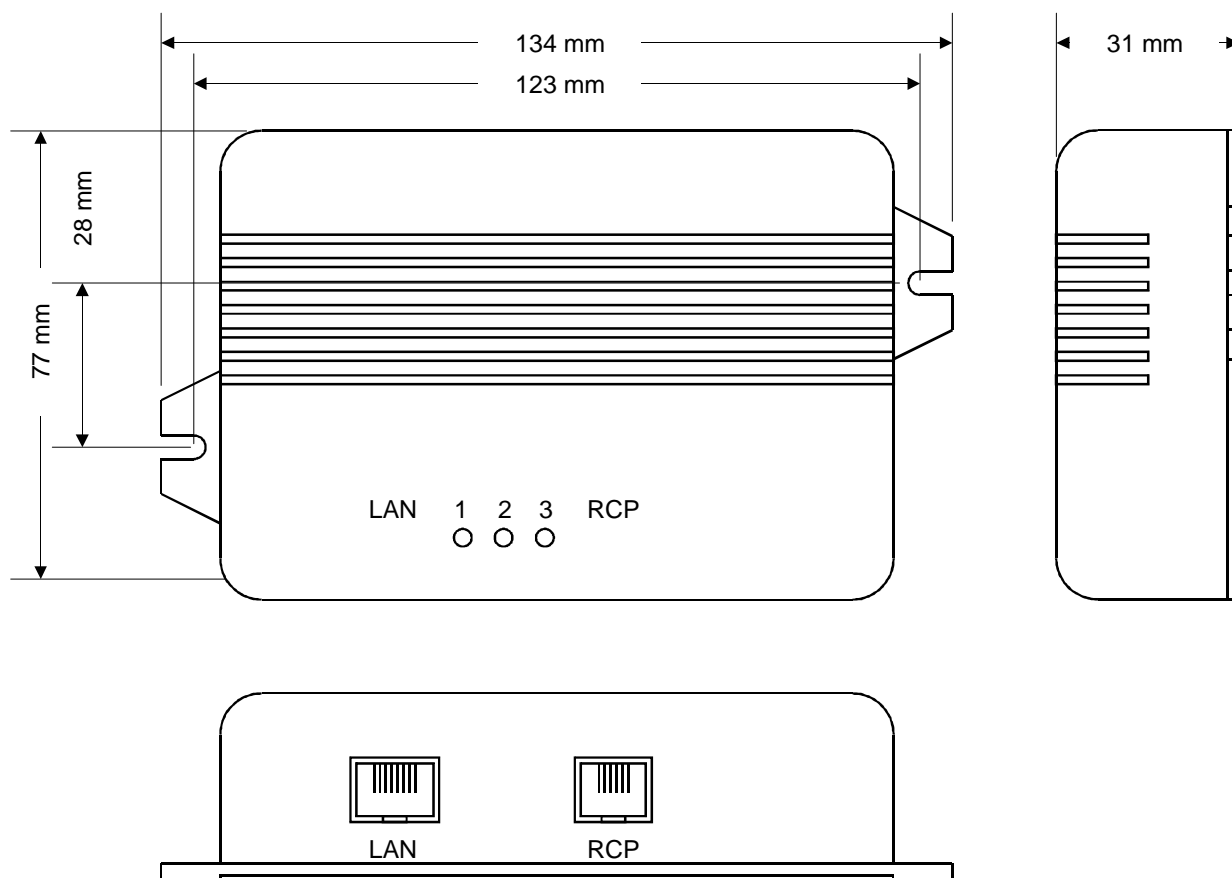
Rysunek 10: Konwerter sieciowy RCP48TS - wymiary główne
