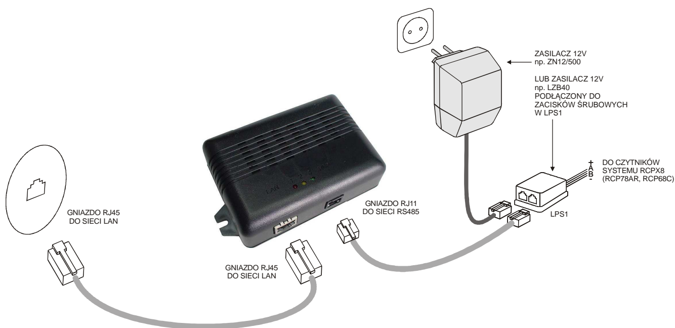
Rysunek 11: Podłączenie konwertera sieciowego RCP48TS
